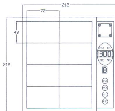
T-AA-300-Front
