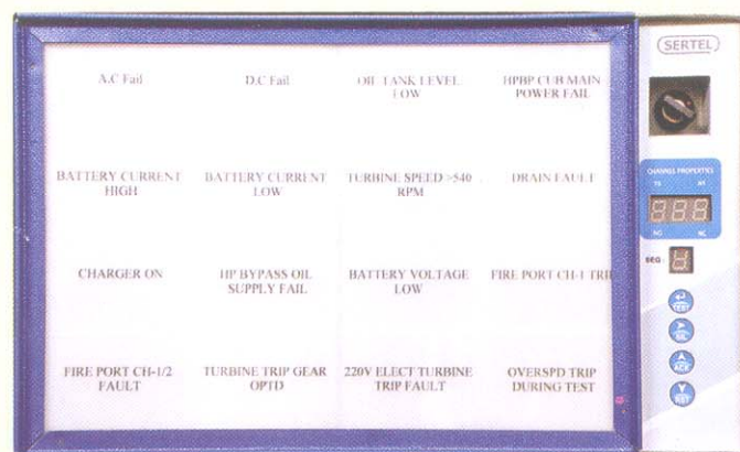
Model : T-AA-300-16-x-x-x
